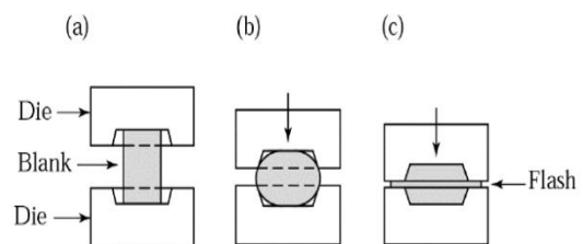
Figure2. Impression die forging
