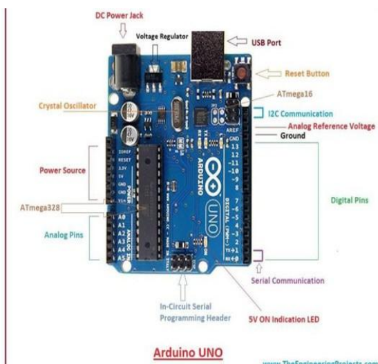
Fig. 2: Arduino UNO.
