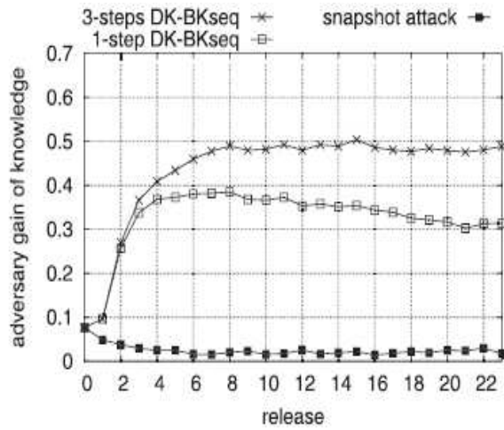
(b) (B,t)-priv.
