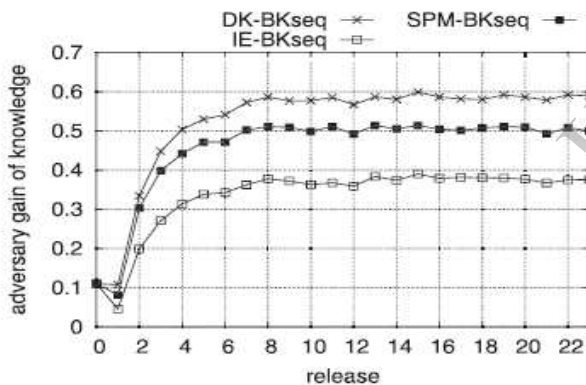
(a) l-div.
