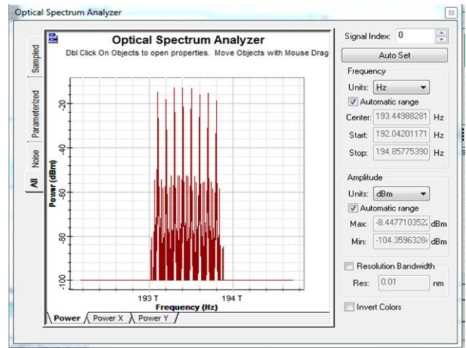
Fig. 4. Input spectrum
