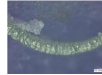
Fig.5 Actual chip morphology
