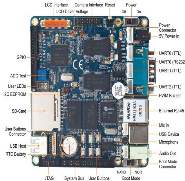
Figure 3.2: Mini 2440 Board
