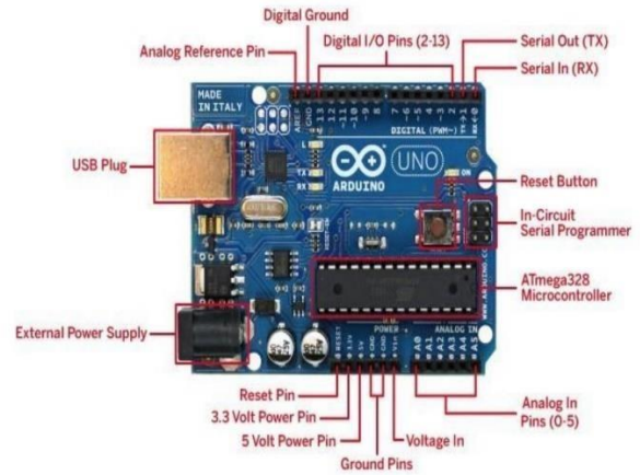
FIG 2. AURDUINO UNO
