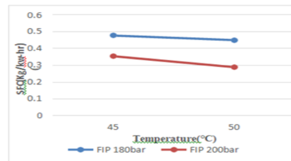
Fig. 8. BSFC (Kg/KW-hr) vs Temperature(°C)
