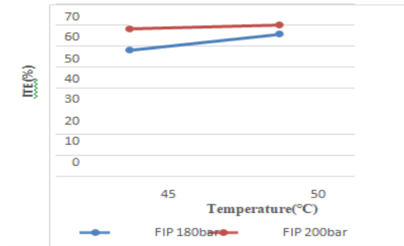
Fig. 6. ITE (%) vs Temperature(°C)
