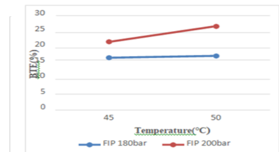
Fig. 7. BTE(%) vs Temperature(°C)
