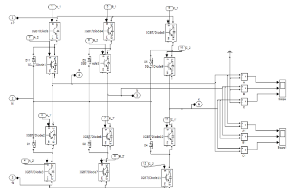
Fig. 5.7 NPC
