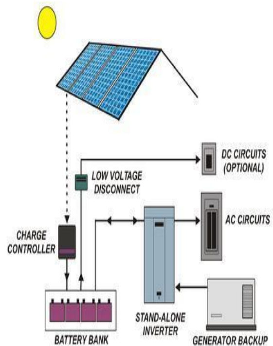
Fig. 3 : Stand alone inverter
